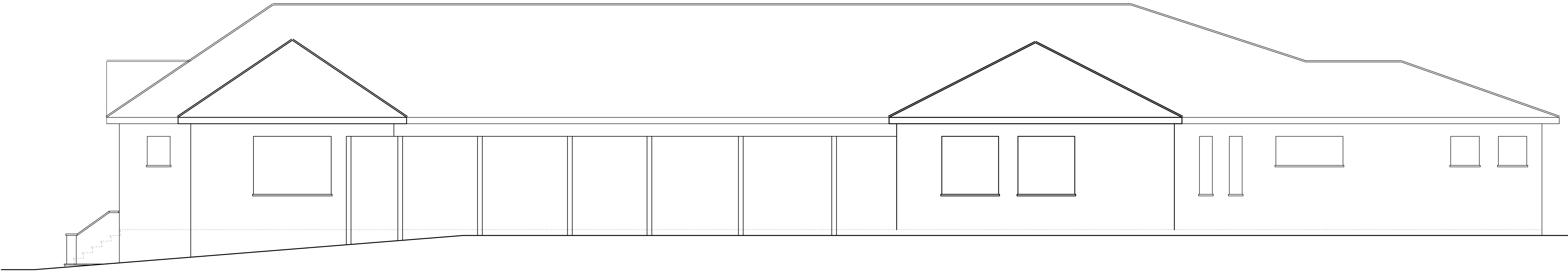
ELEVACIÓN ORIENTE ESCALA: 1/50
